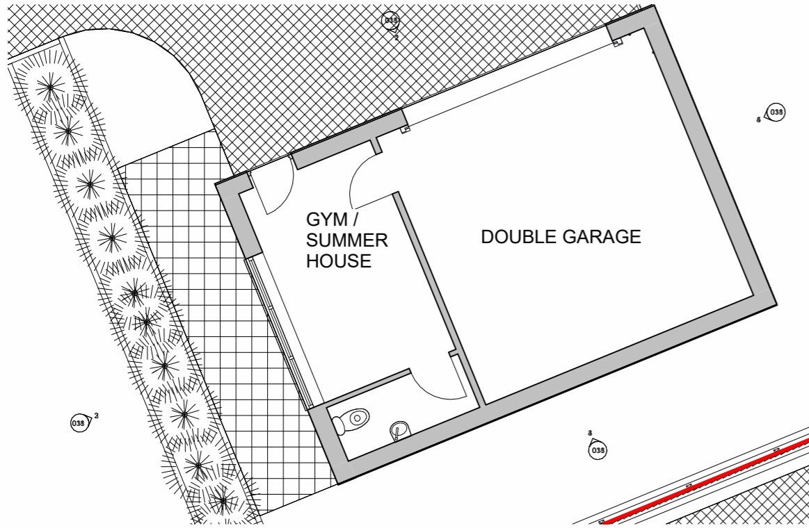
1 Plot 2 Garage Plan 1 : 100
