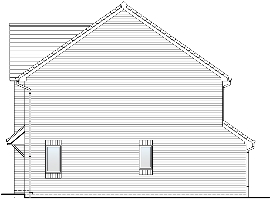
Right Elevation
