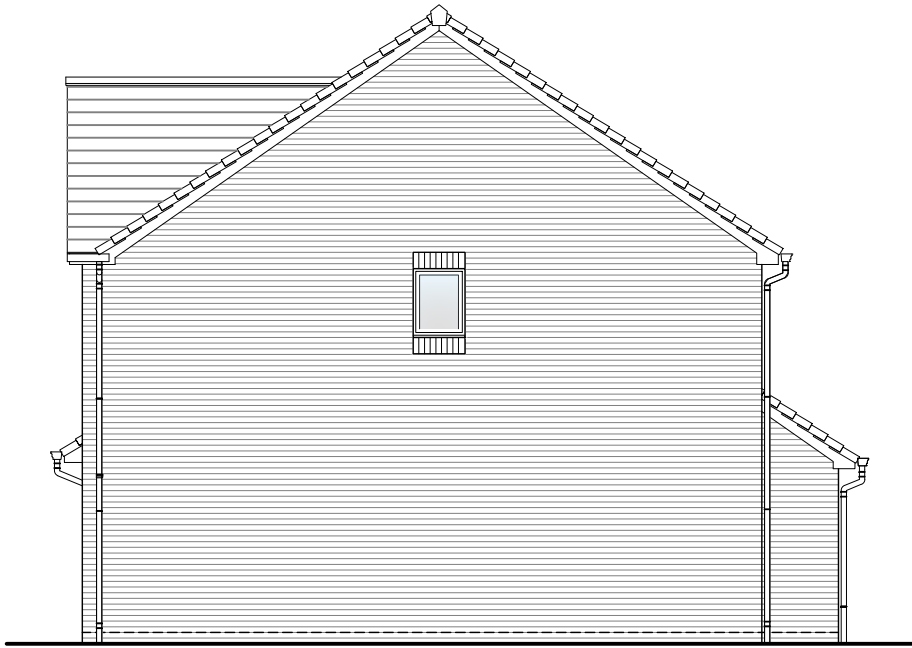
Right Elevation
