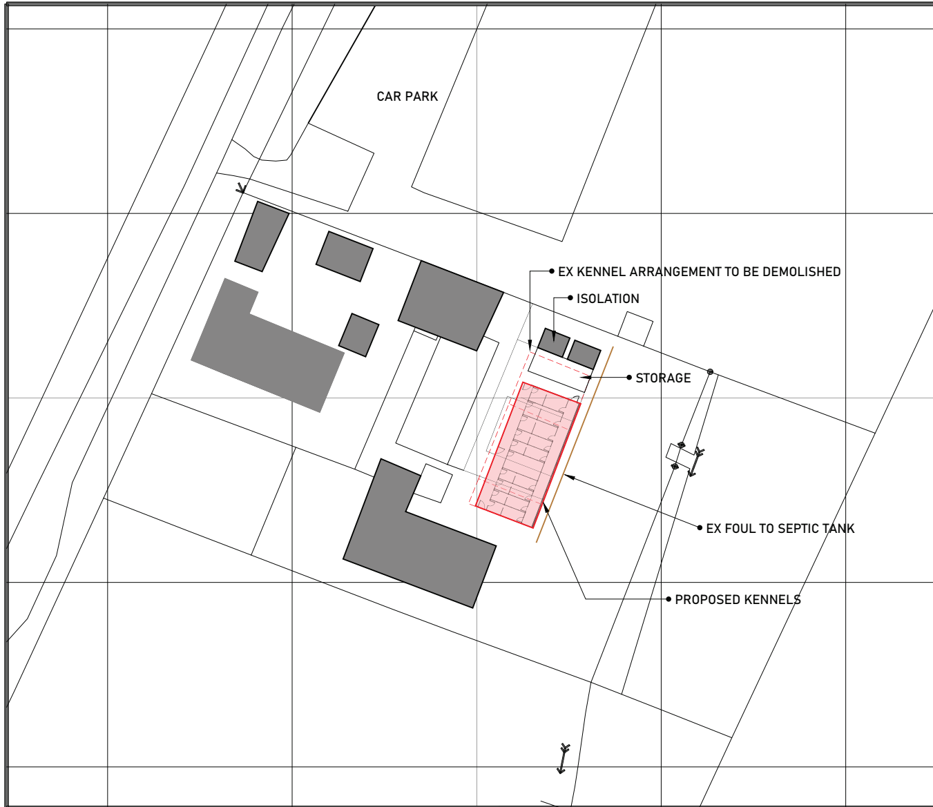
SITE PLAN 1:500
