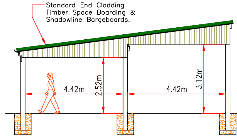
End Elevation
