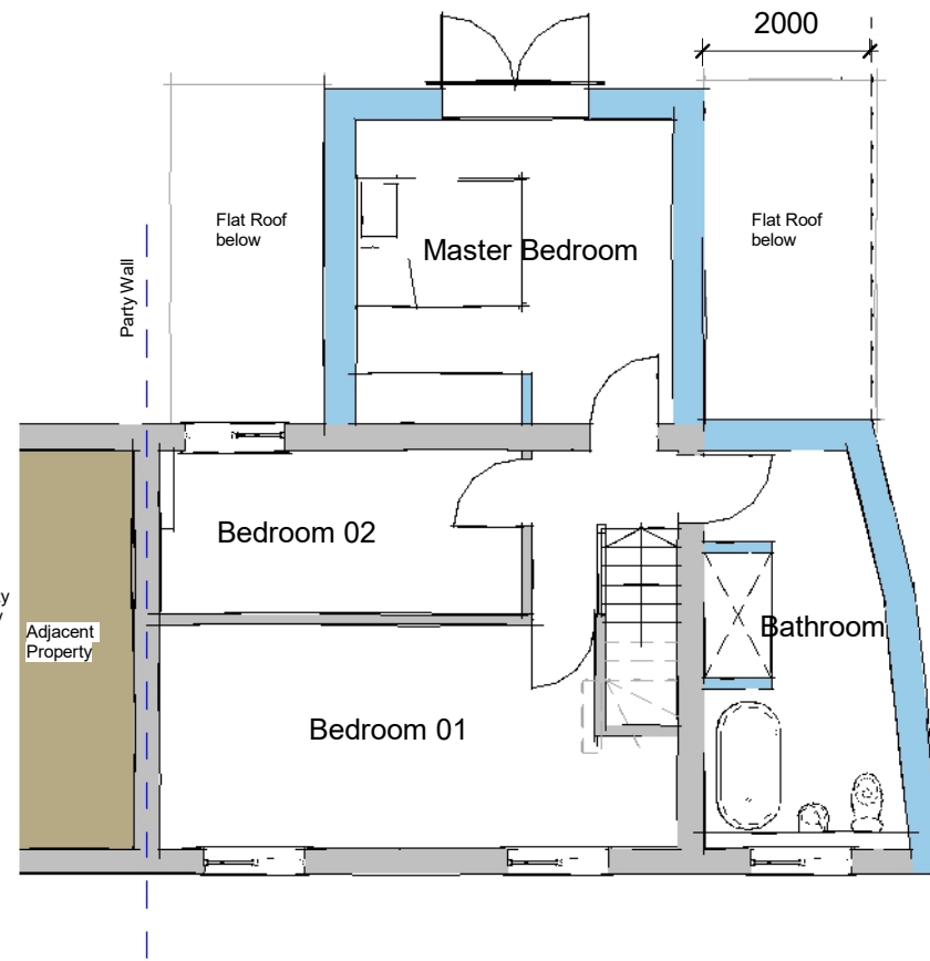
First 1 : 100
