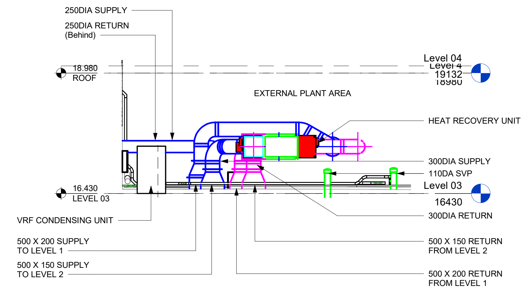
3 Section 14 1 : 50
