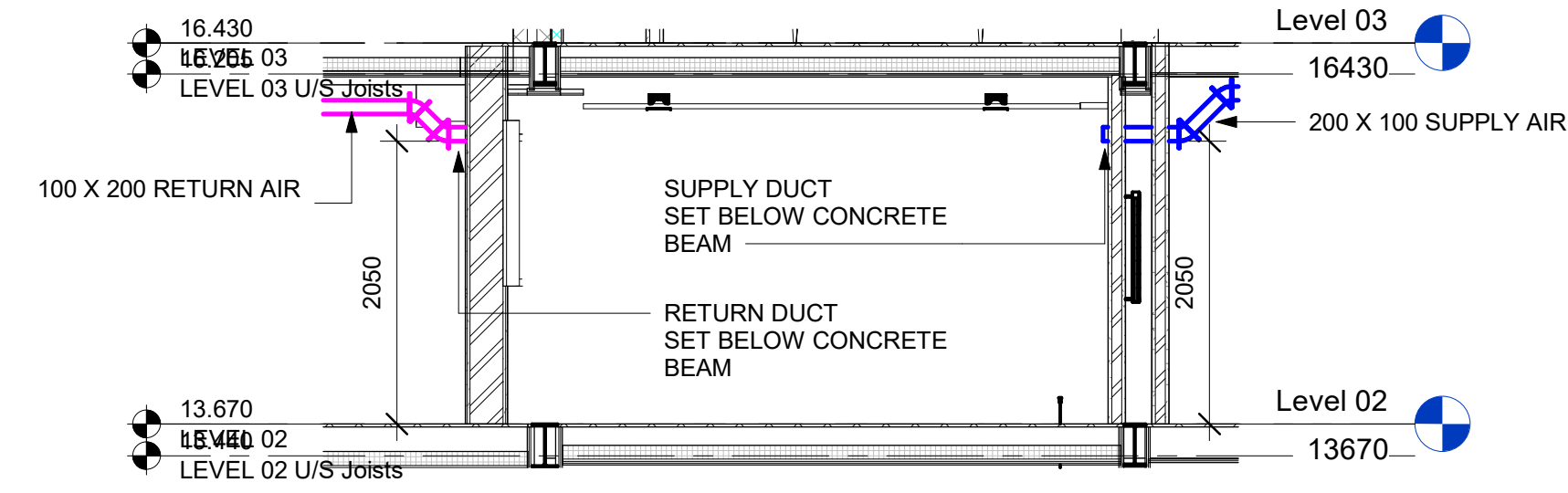
5 Section 10 1 : 50
