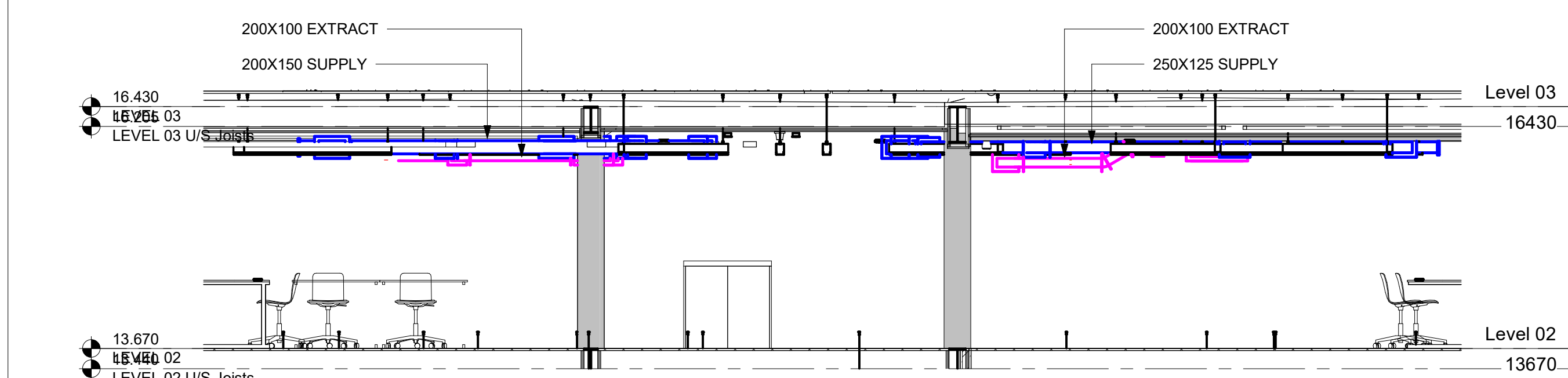
2 Section 6 1 : 50
