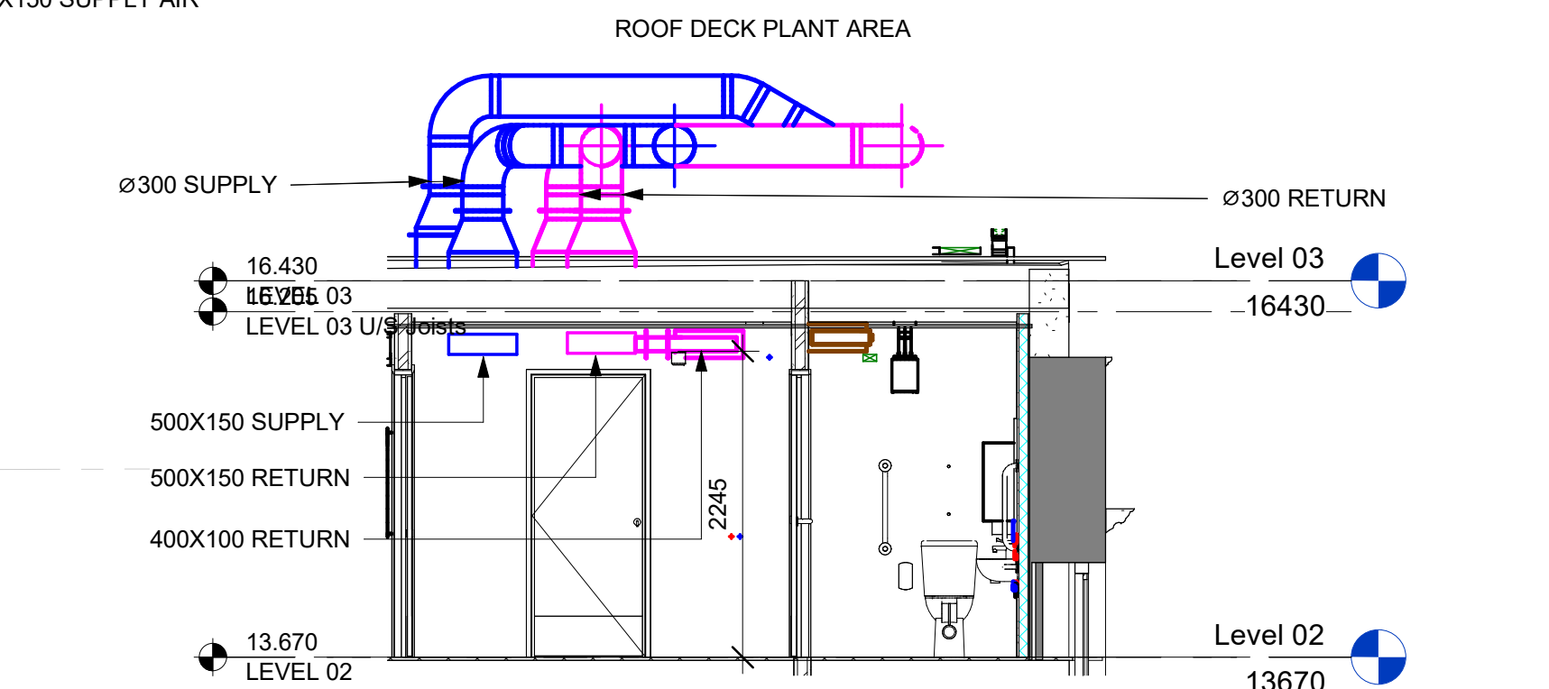
3 Section 7 1 : 50
