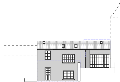
6 A101 SCALE: 1:100
