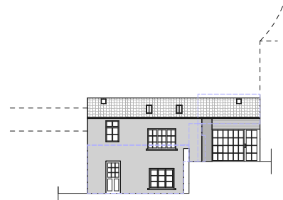
3 A101 SCALE: 1:100
