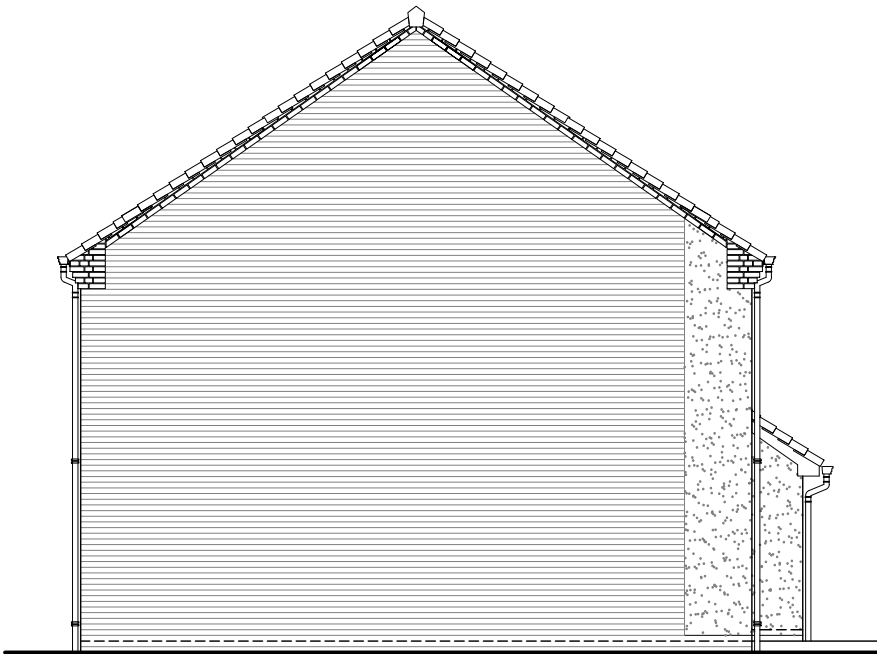
Right Elevation
