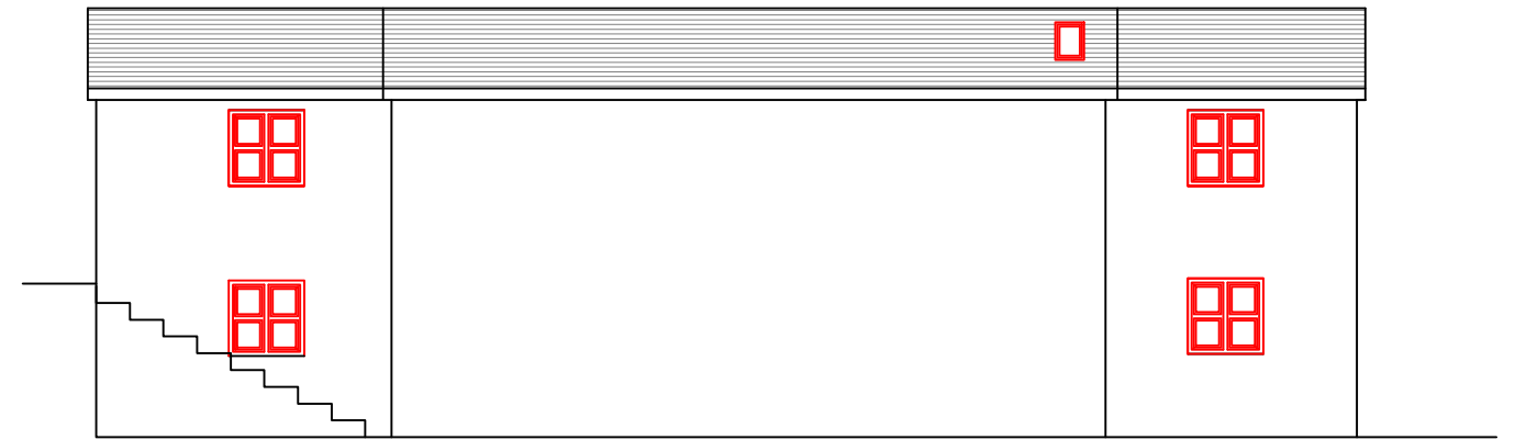
EXISTING REAR ELEVATION SCALE: 1:100 @ A3
