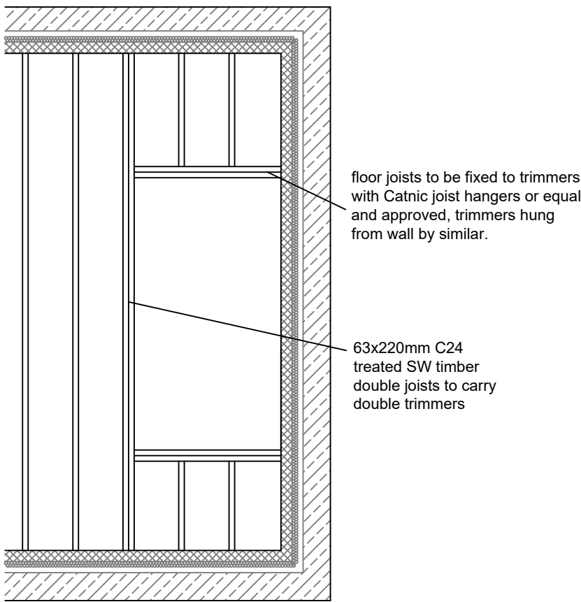
Trimmer Plan
