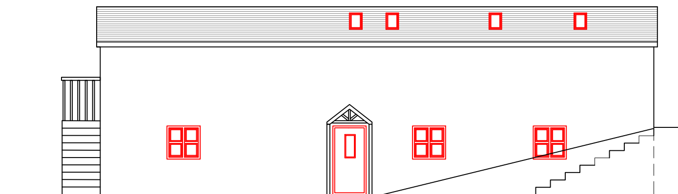
EXISTING FRONT ELEVATION SCALE: 1:100 @ A3
