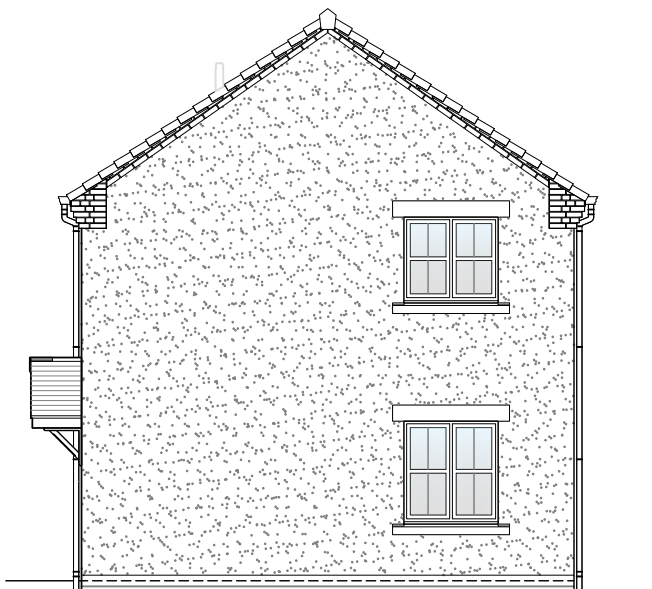
Right Elevation
