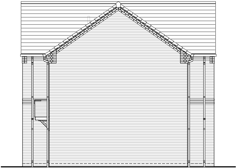
Right Elevation
