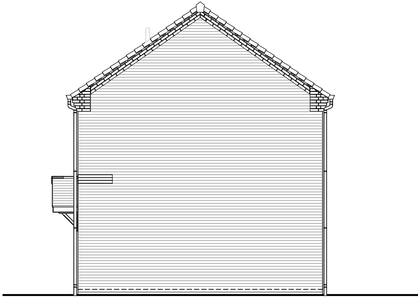
Right Elevation
