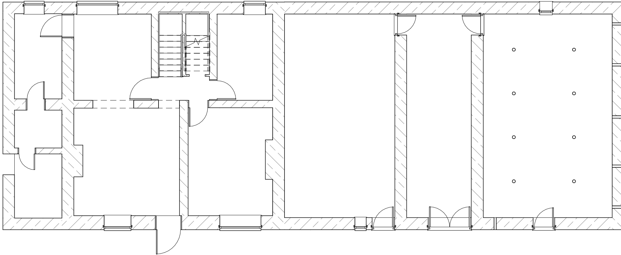
1 Level 0 - Callout 2 1 : 100
