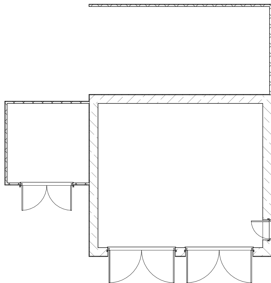
1 Level 0 - Callout 1 1 : 100
