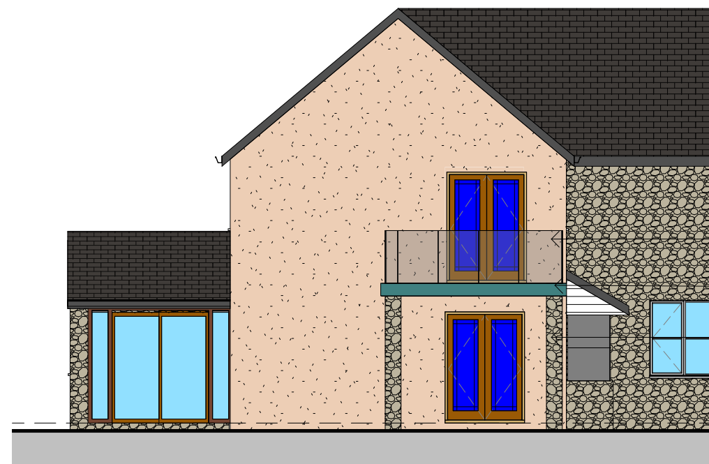
1 East 1 : 100
