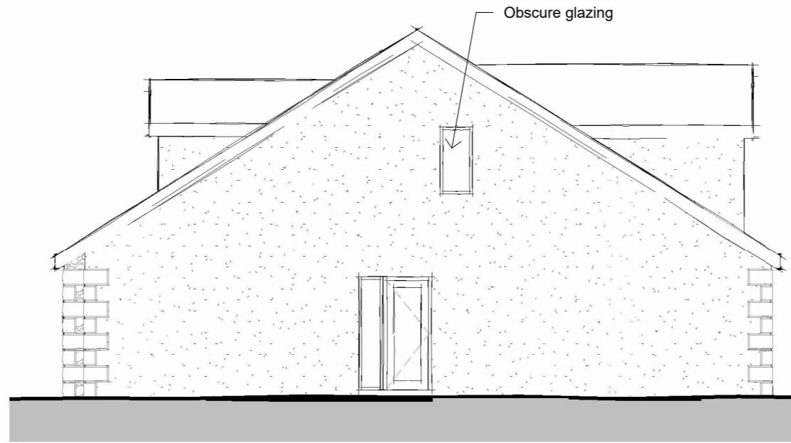
Side Elevation 01 1 : 100
