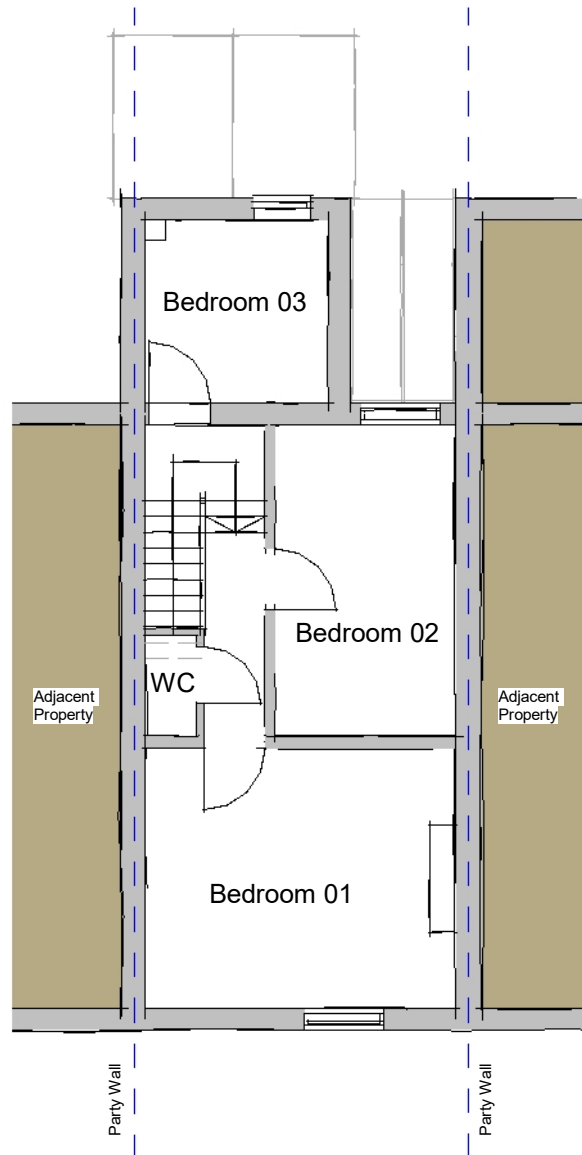
First 1 : 100
