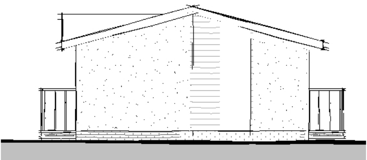
Side Elevation 01 1 : 100
