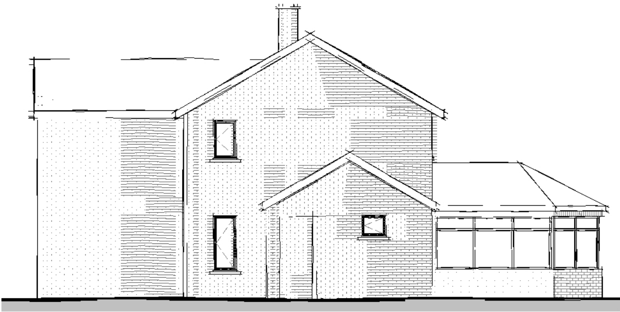
Side Elevation 01 1 : 100
