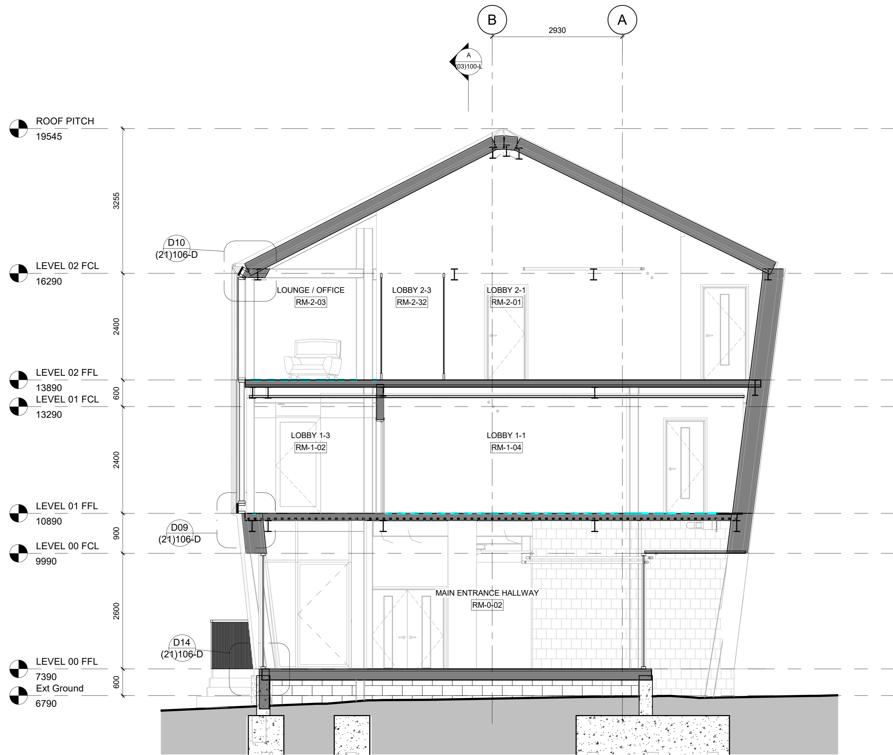
SECTION CC 1 : 50
