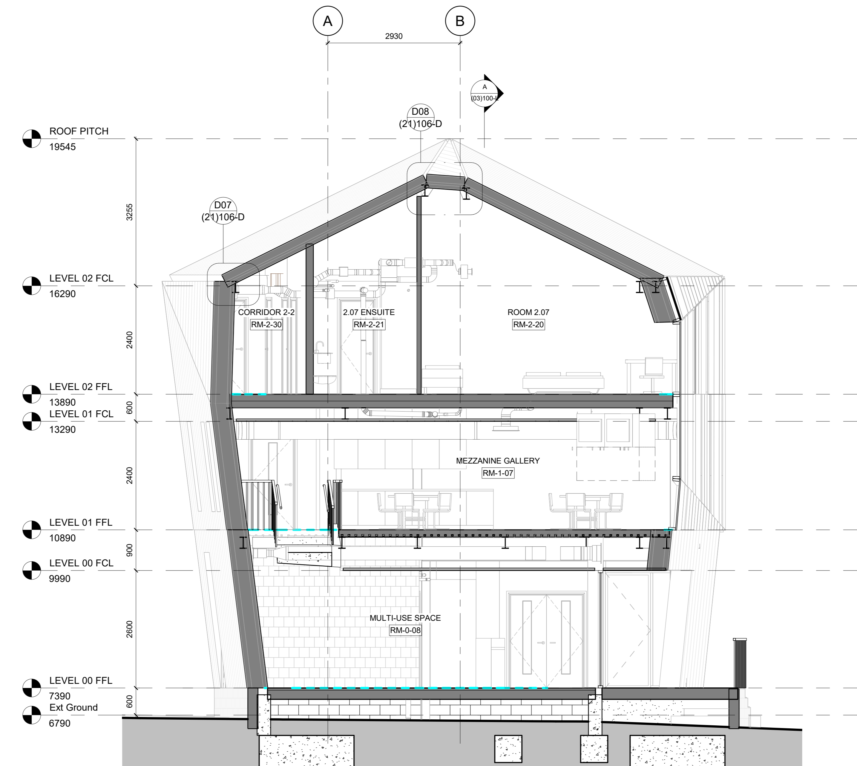
SECTION DD 1 : 50
