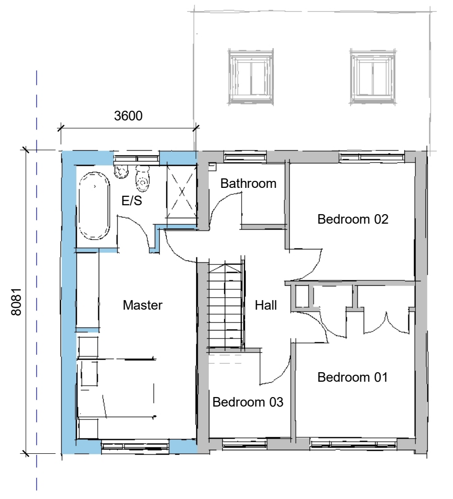
First 1 : 100
