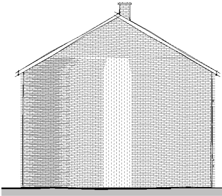
Side Elevation 01 1 : 100
