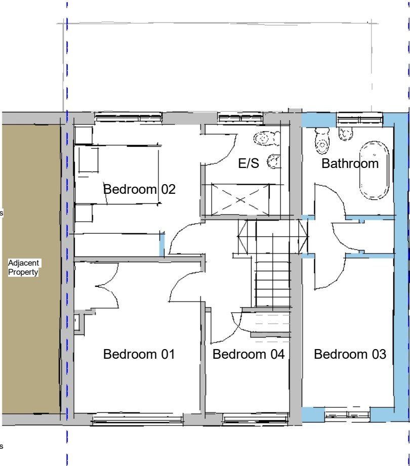
First 1 : 100
