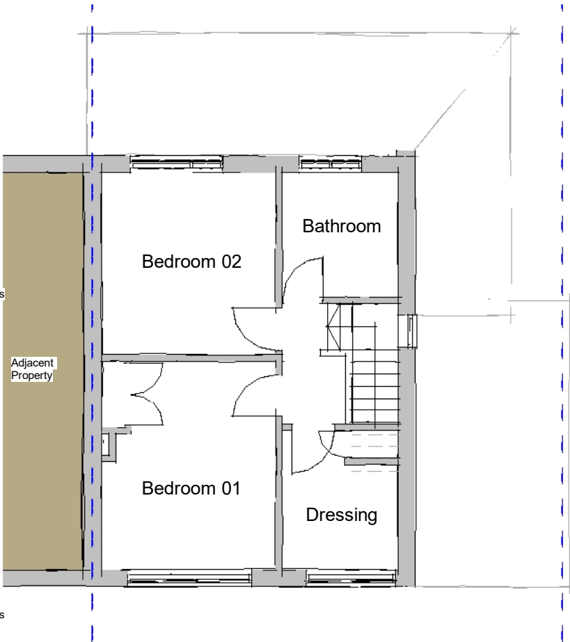
First 1 : 100
