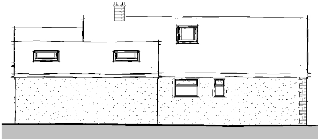
Side Elevation 01 1 : 100
