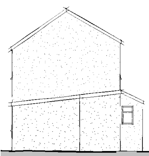
Side Elevation 01 1 : 100
