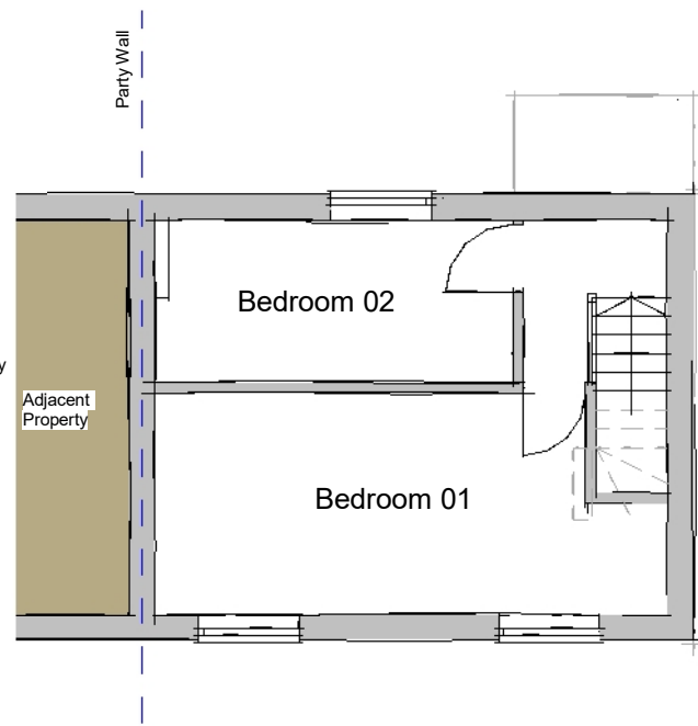
First 1 : 100
