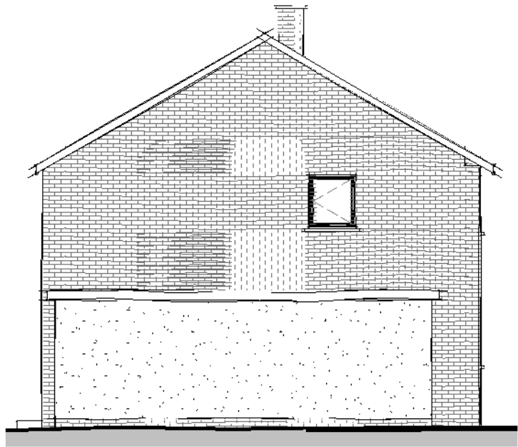
Side Elevation 01 1 : 100
