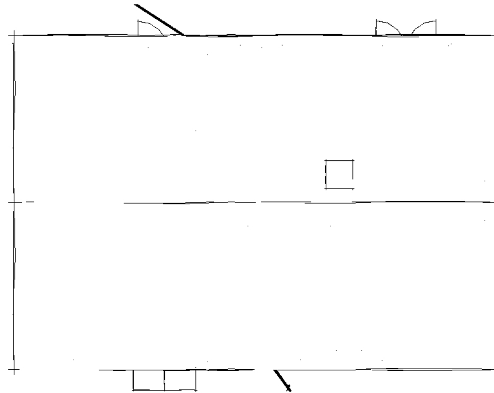
Roof Plan 1 : 100
