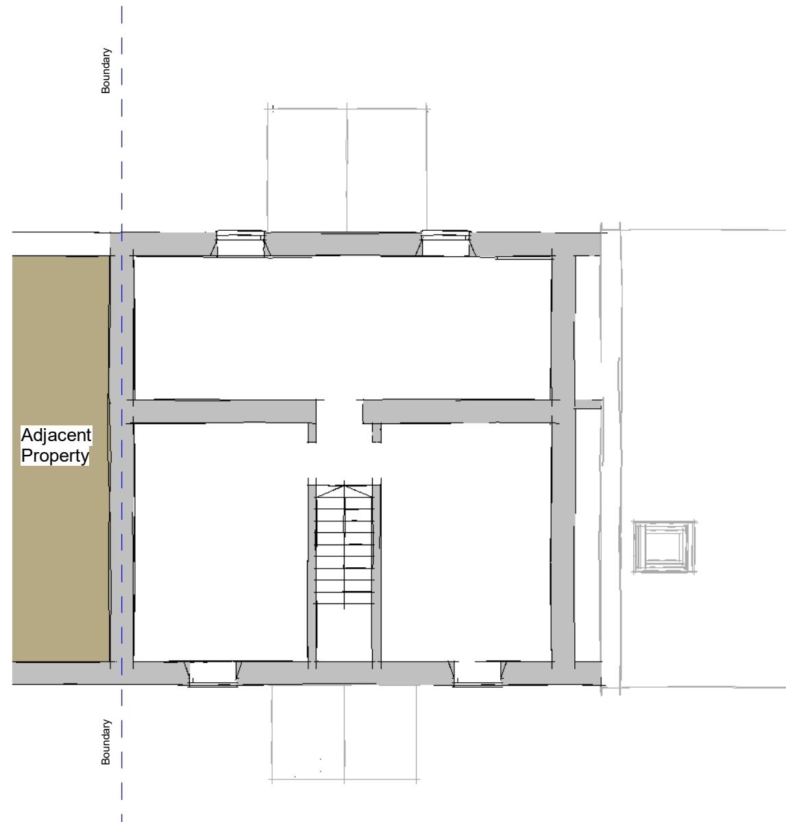
First 1 : 100
