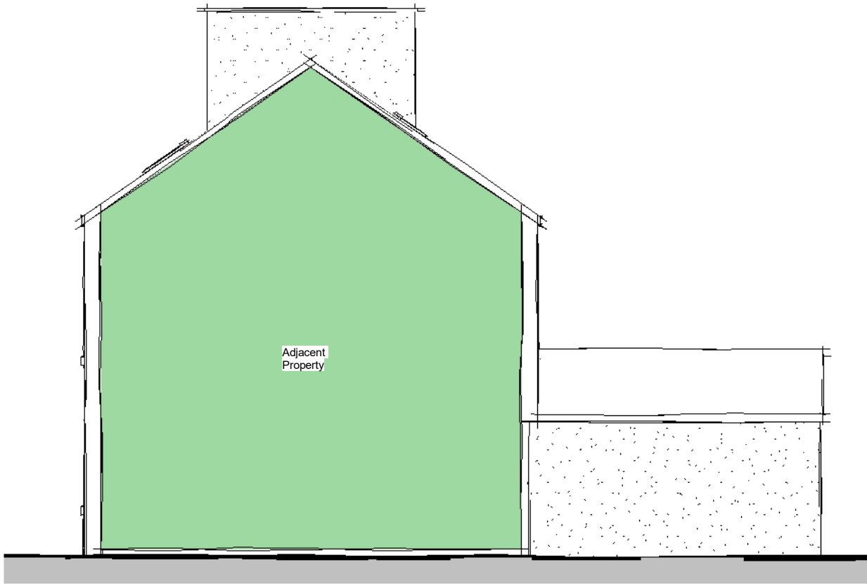
Side Elevation 01 1 : 100
