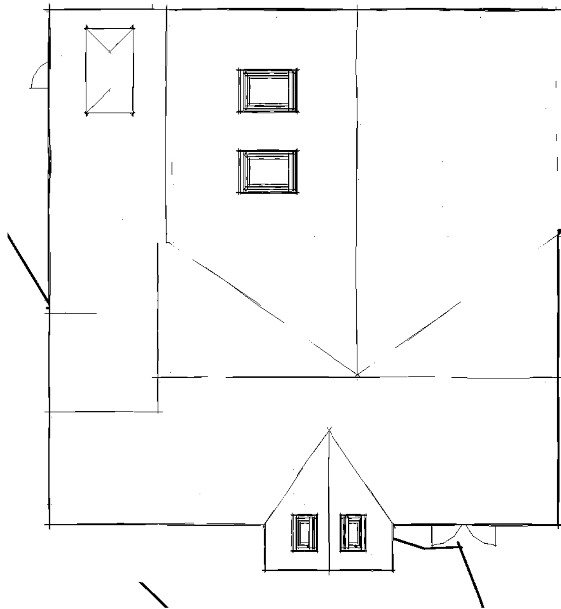
Roof Plan 1 : 100
