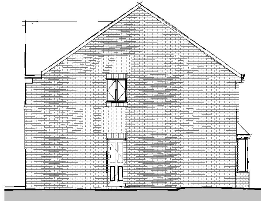
Side Elevation 01 1 : 100
