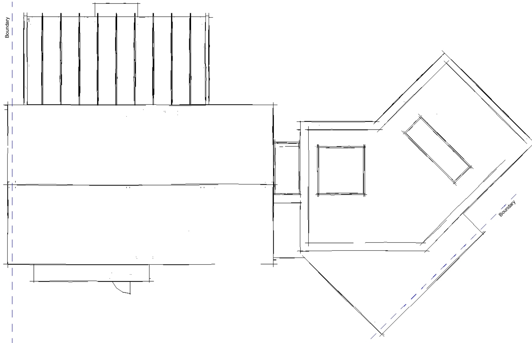
Roof Plan 1 : 100
