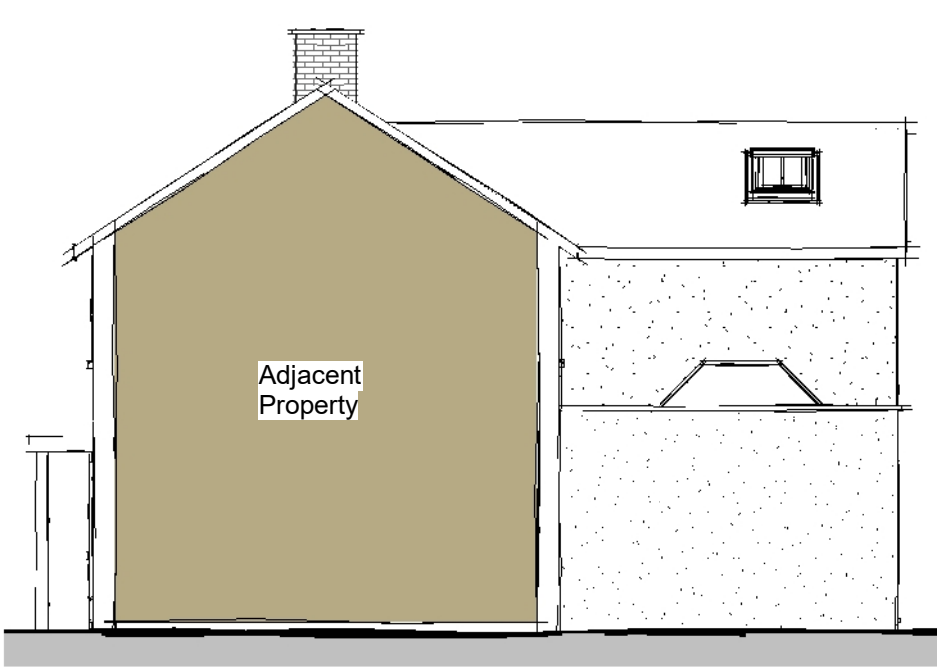
Side Elevation 01 1 : 100
