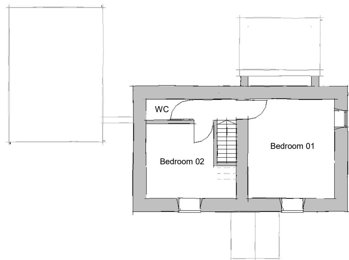
First 1 : 100
