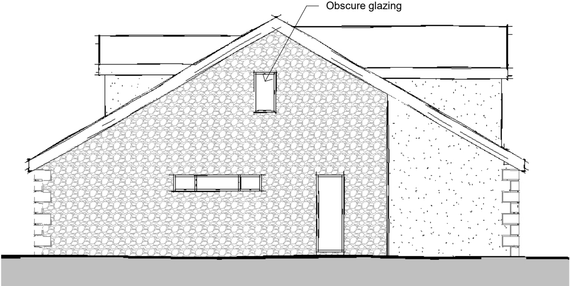
Side Elevation 01 1 : 100
