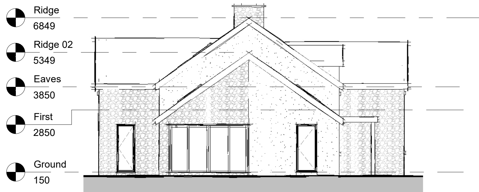
Side Elevation 01 1 : 100
