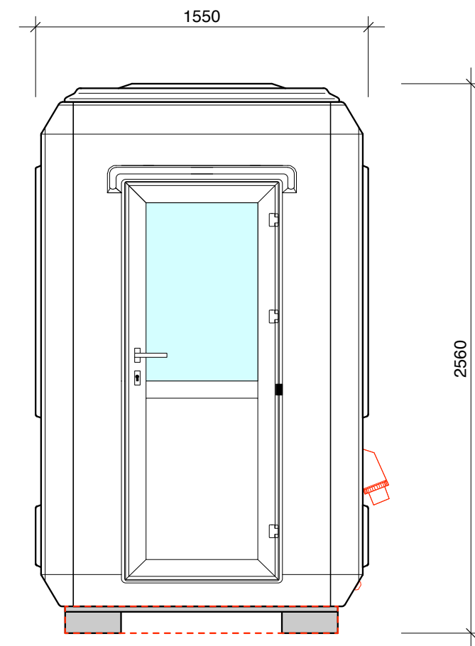
ELEVATION 'C'
