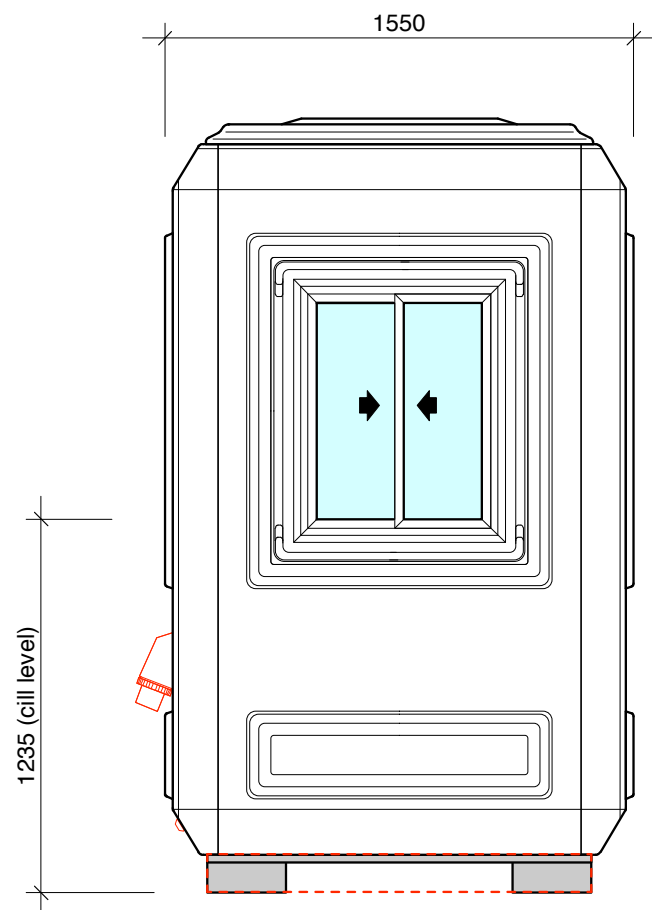
ELEVATION 'B'
